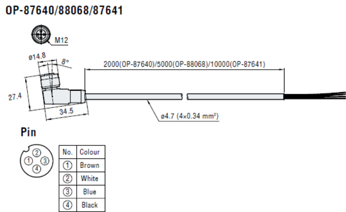
OP-87640_88068_87641_dimension_01.gif
