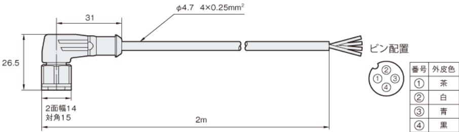
op_87276_dimension_01.gif
