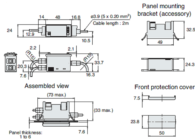
AP-V85_V87_panelcutout_dimension_01.gif
