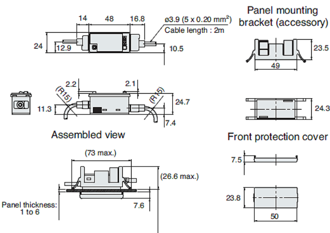
AP-V85_V87_panelcutout_dimension_01.gif
