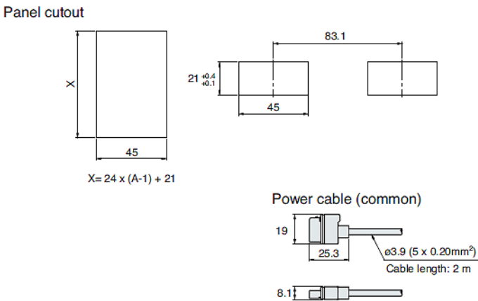
AP-V85_V87_panelcutout_dimension_01.gif
