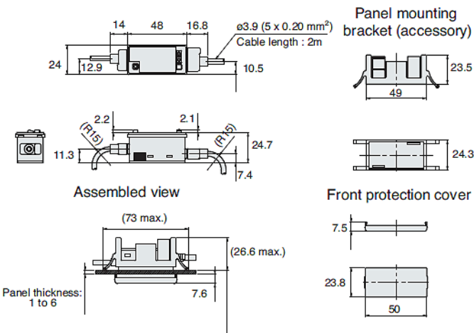
AP-V85_V87_panelcutout_dimension_01.gif
