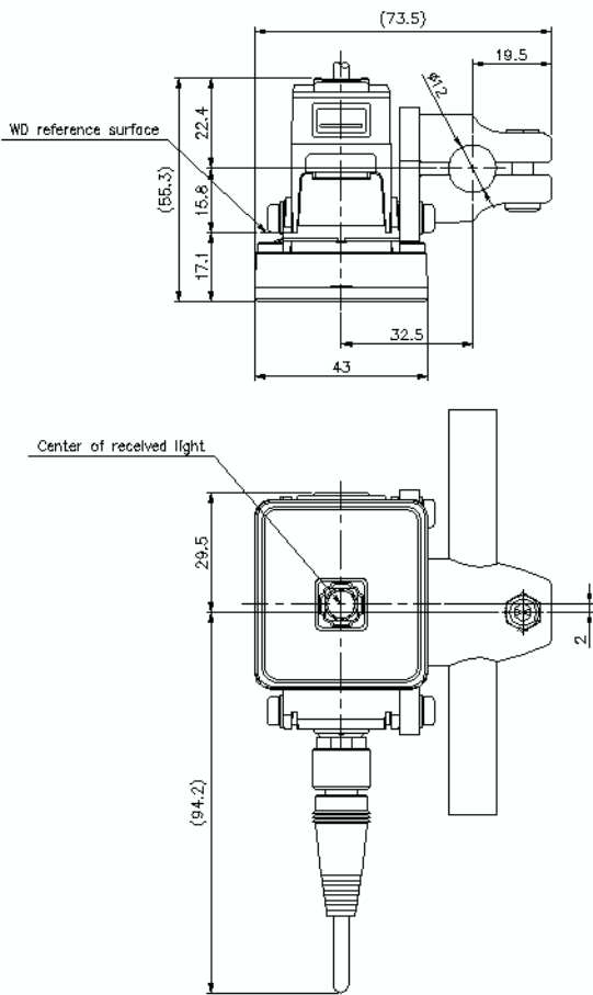
aib_d16b_88116_dimension_01.gif
