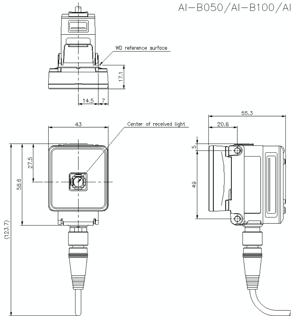
aib050-160_d16b_dimension_01.gif
