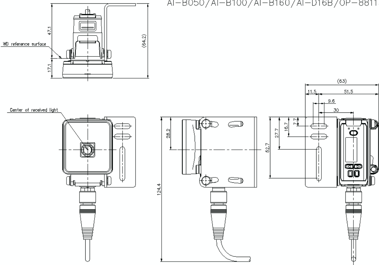
aib_d16b_88115_dimension_01.gif
